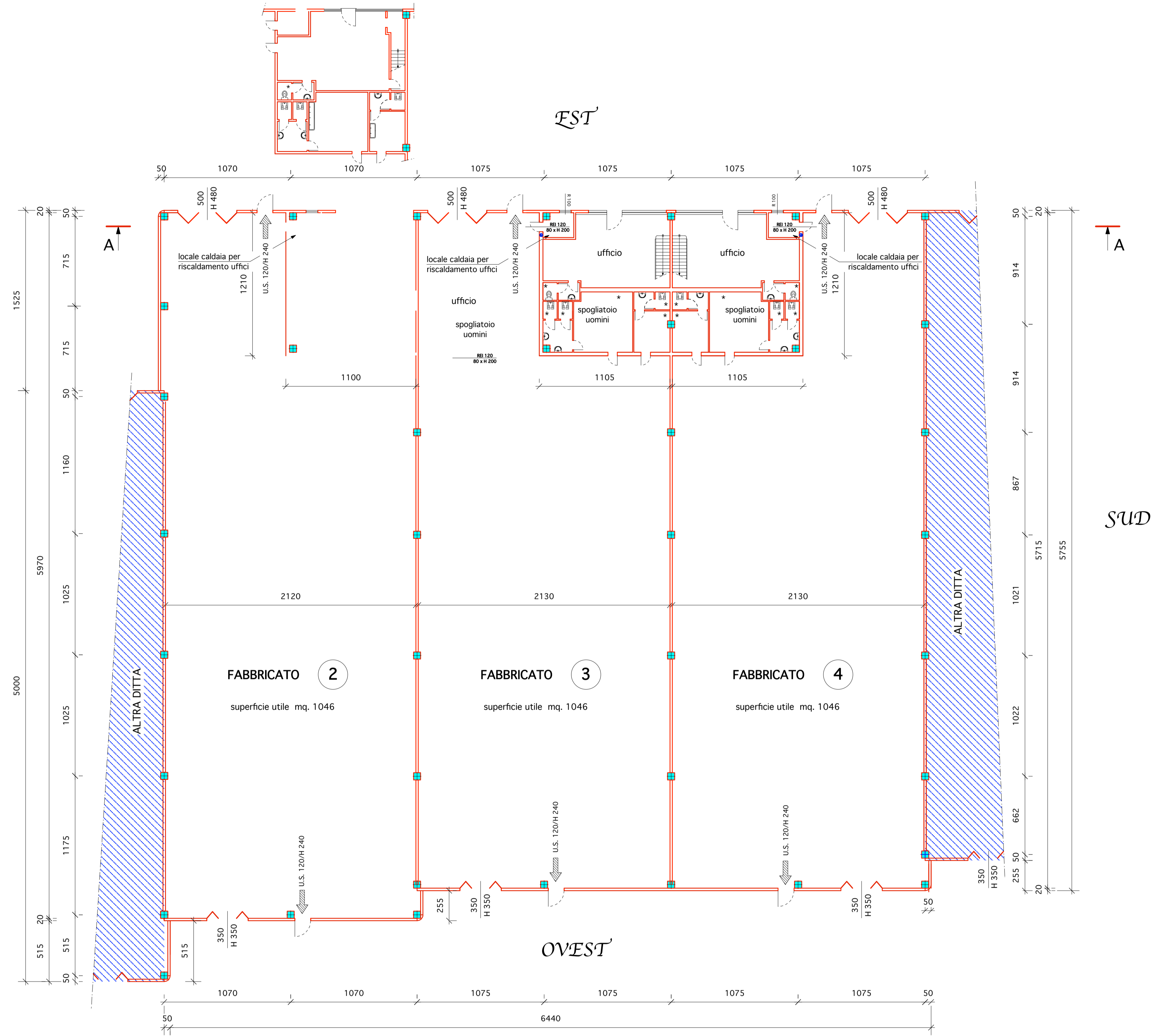
PIANTA CAPANNONI
