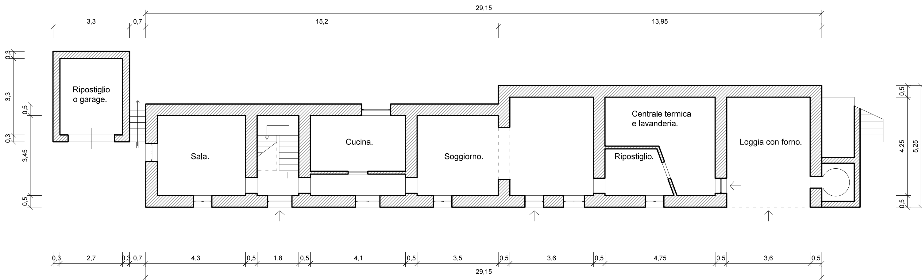
PIANTA PIANO TERRENO.
