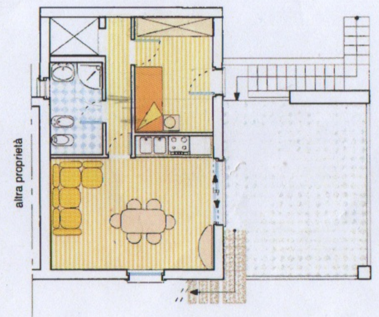
PIANO PRIMO Scala 1:200
