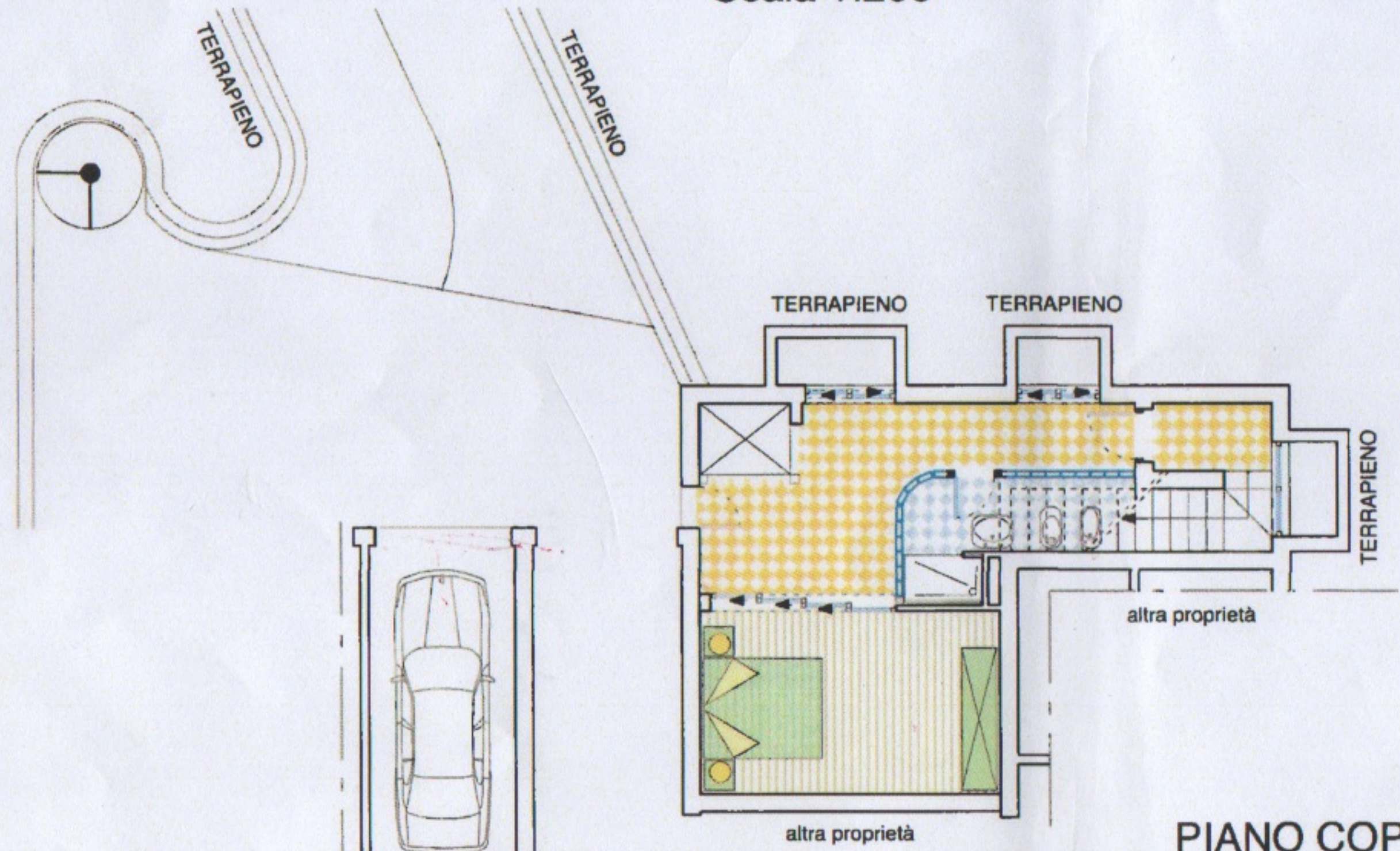
PIANO INTERRATO Scala 1:200
