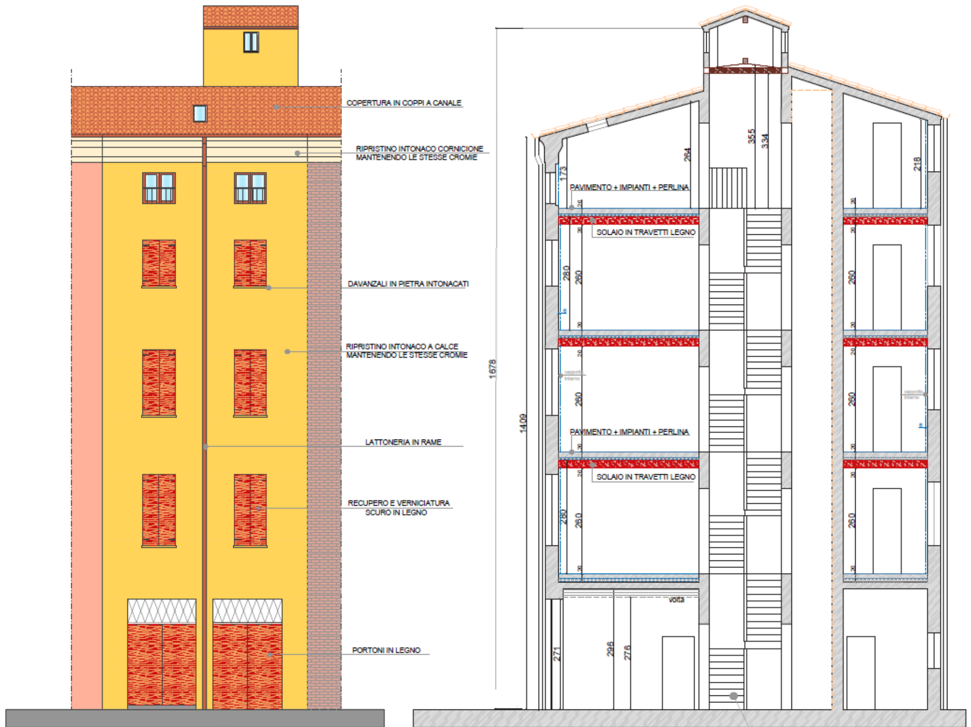
SEZIONE A-A'
