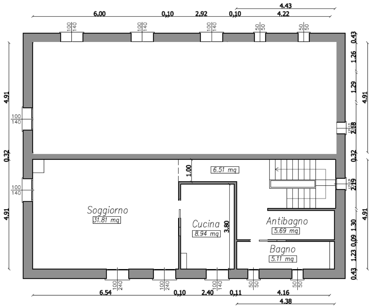
Piano primo
