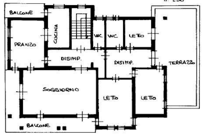
PIANO PRIMO h. 290
