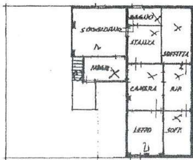
PIANO SECONDO N. 1,00 in scala
