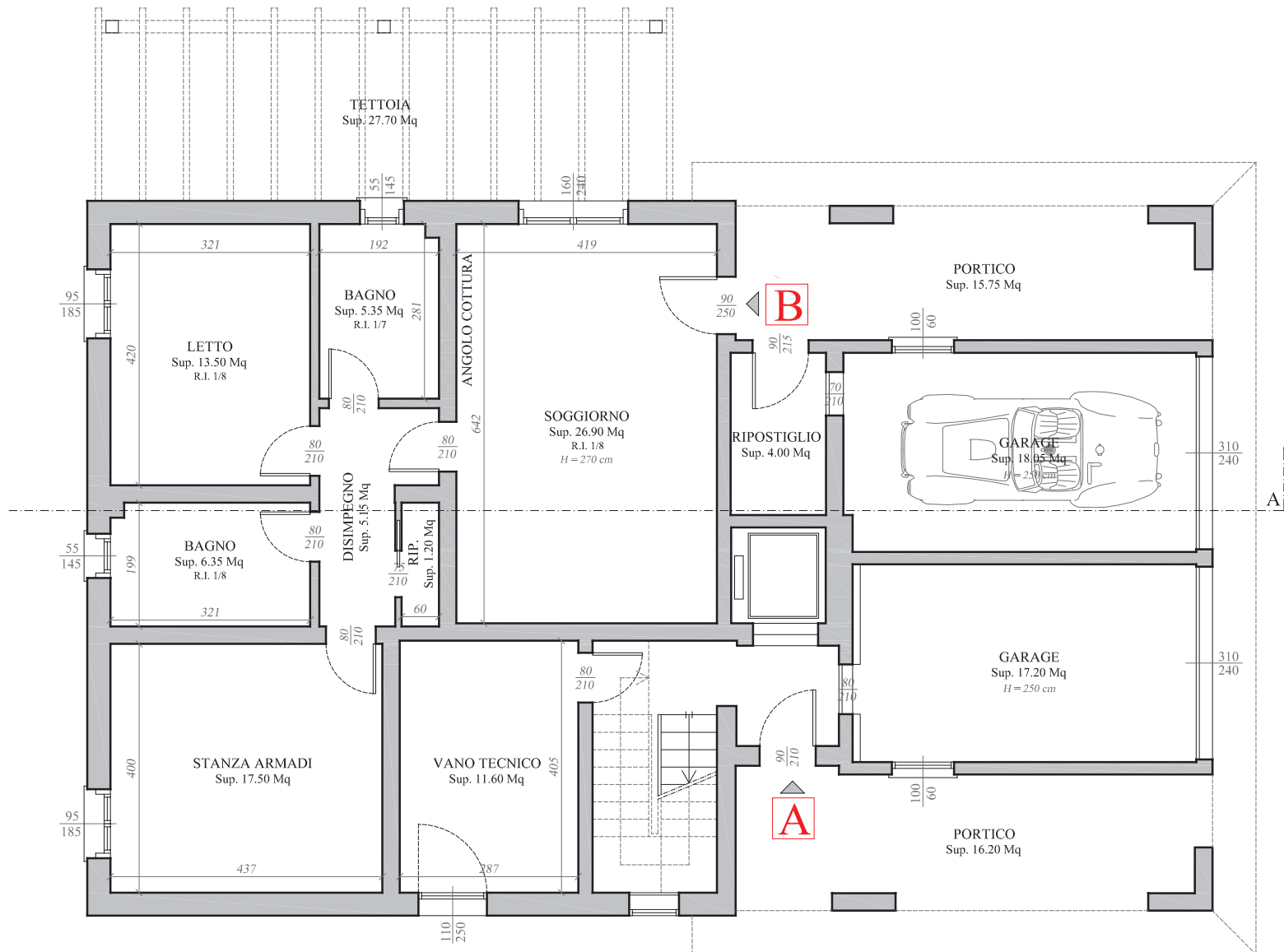
PROGETTO PIANTA PIANO TERRA Scala 1:100
