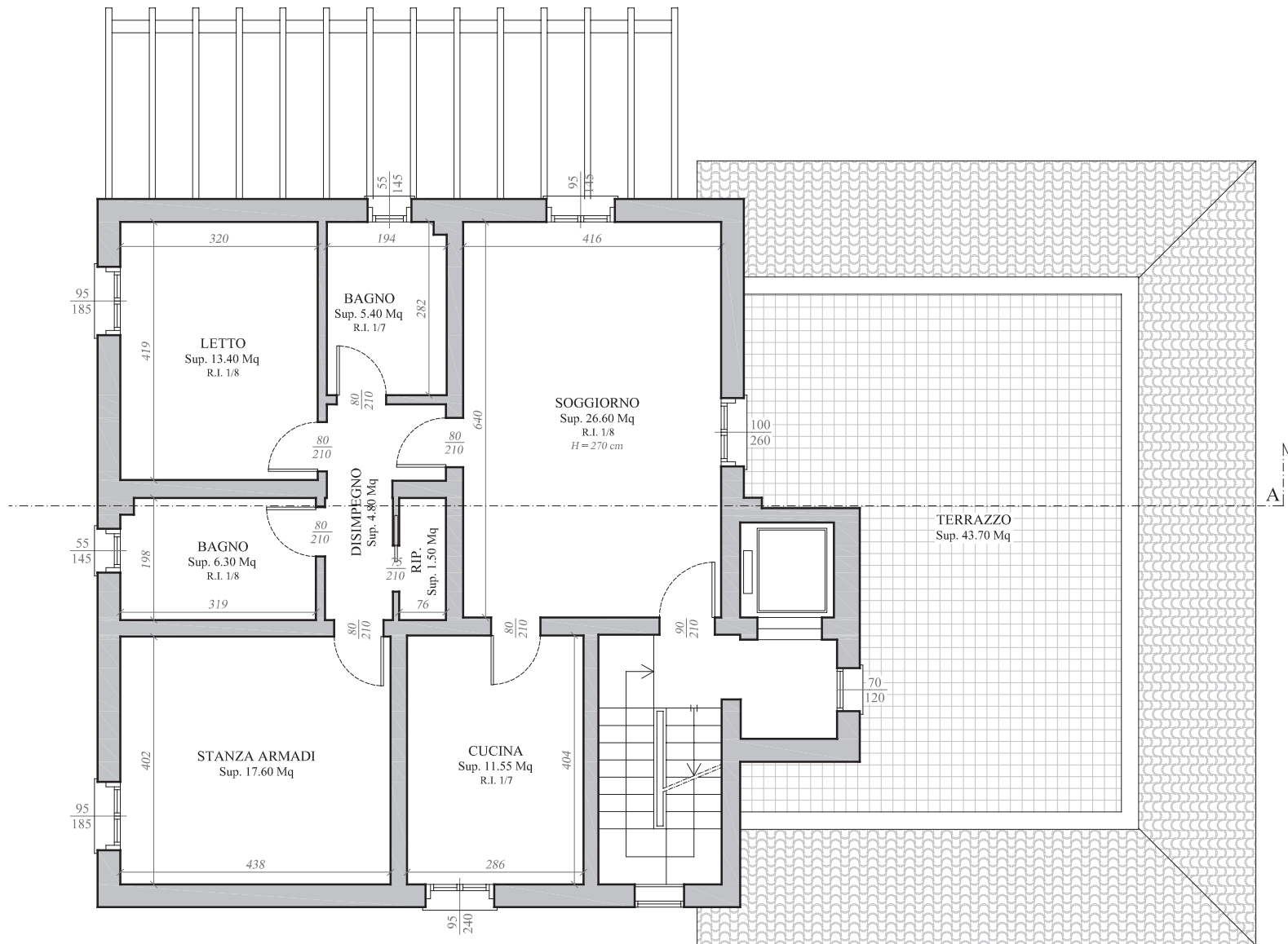
PROGETTO PIANTA PIANO PRIMO Scala 1:100
