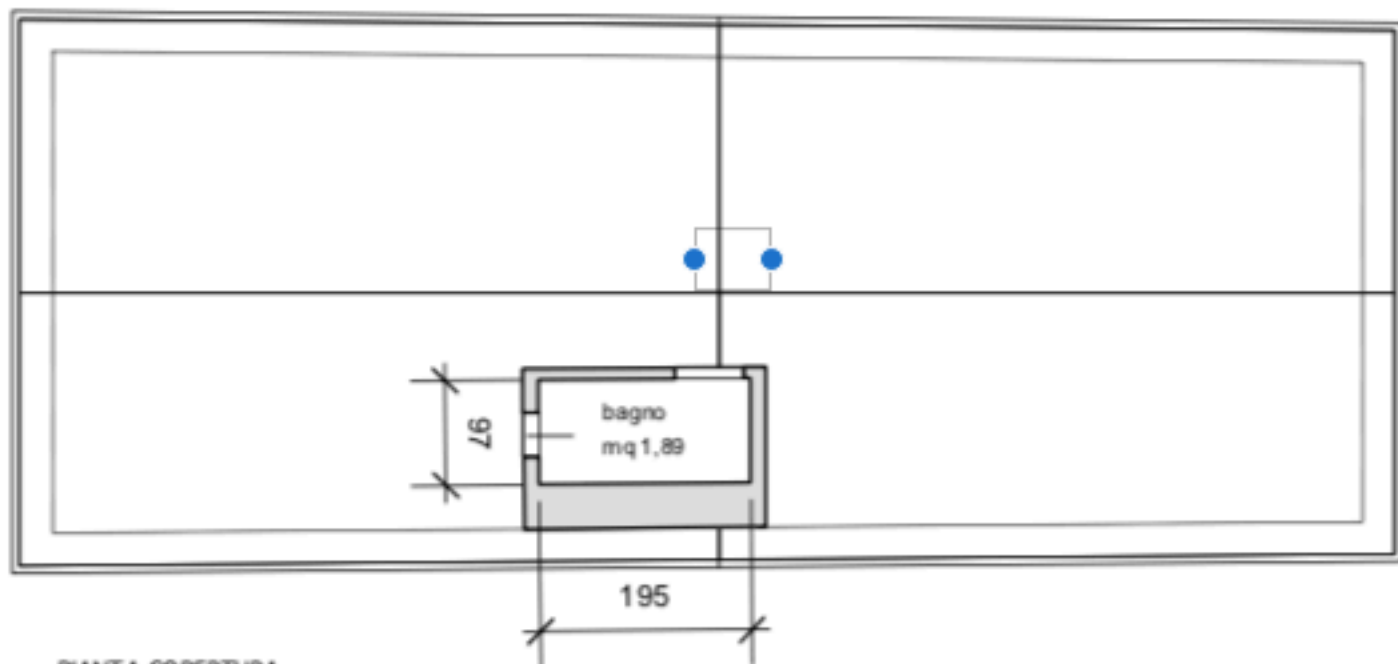
PIANTA COPERTURA
