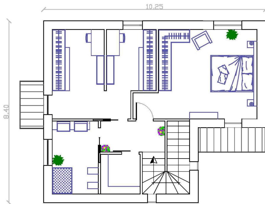
PIANO PRIMO H= 2.80 Mt.
