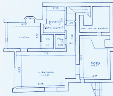
PIANTA PIANO SEMINTERRATO
