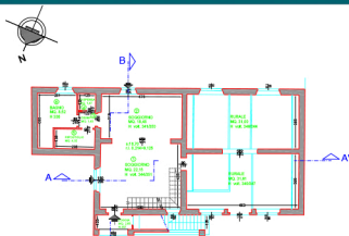
PIANTA PIANO TERRA SCALA 1:100
