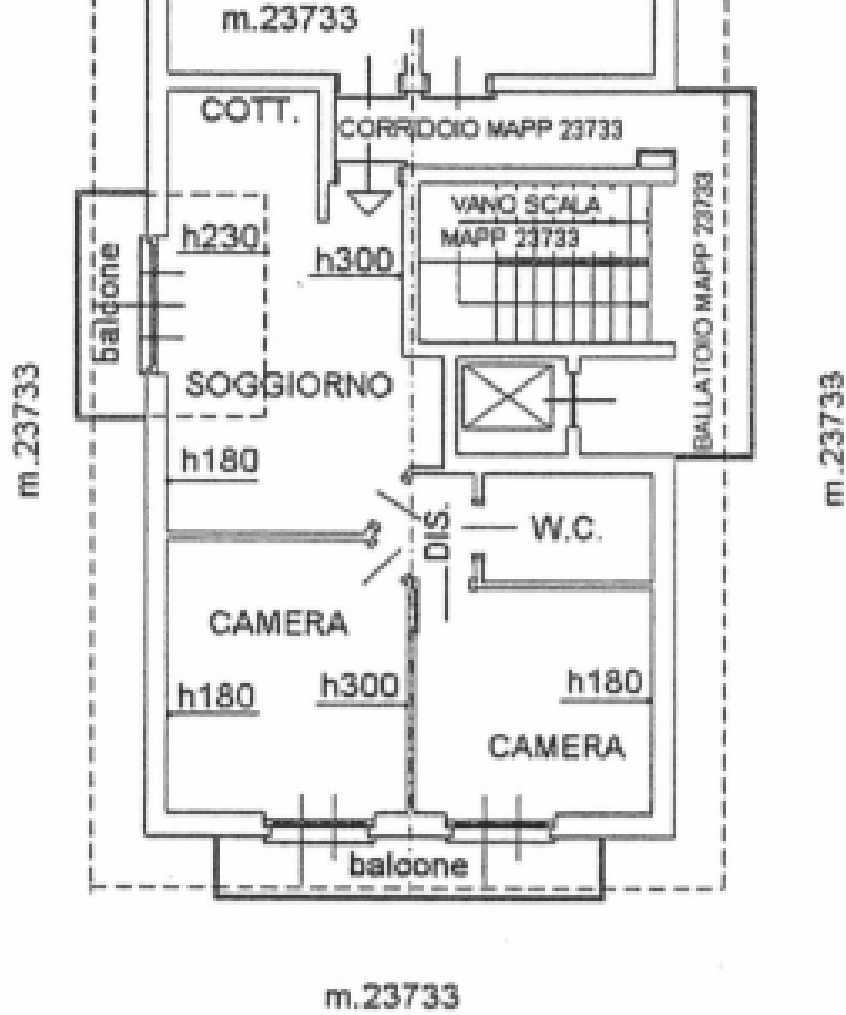
PIANO TERZO (SOTTOTETTO) h.=240cm.
