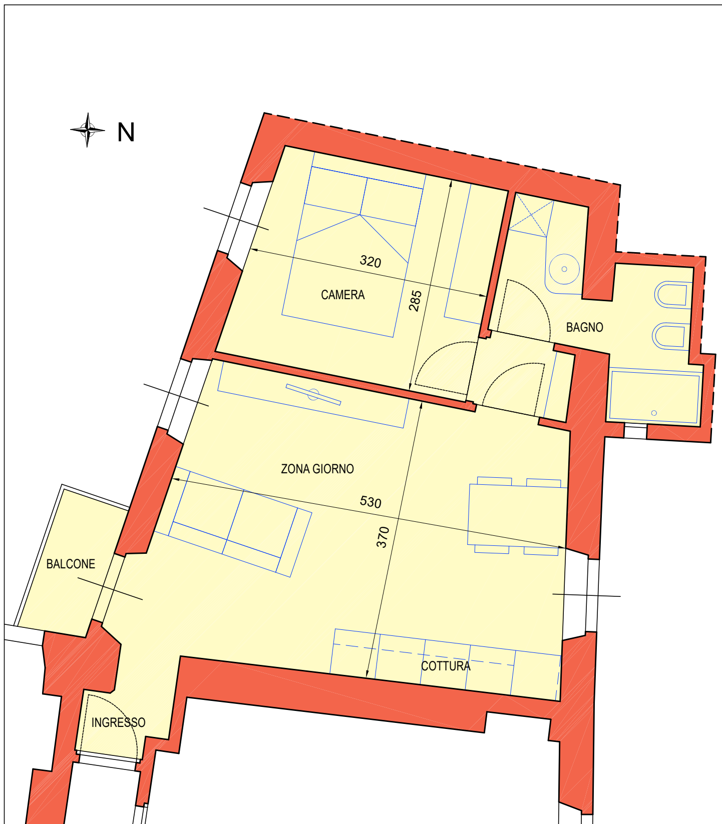
ALLOGGIO 01 - PIANO SECONDO - SCALA 1:50
