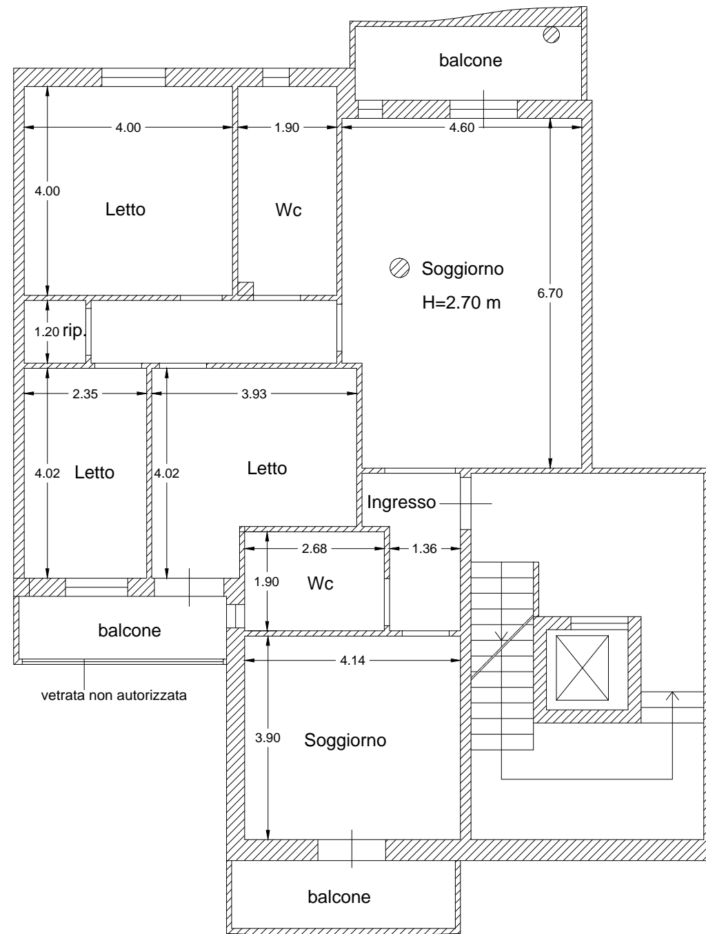
PIANTA APPARTAMENTO PIANO PRIMO_INT.4 scala 1:100
