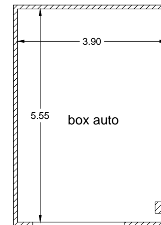
PIANTA BOX AUTO N. 35 PIANO INTERRATO scala 1:100
