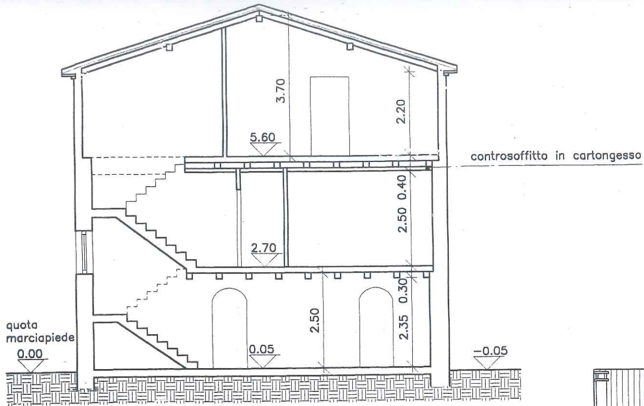
SEZIONE A-A
