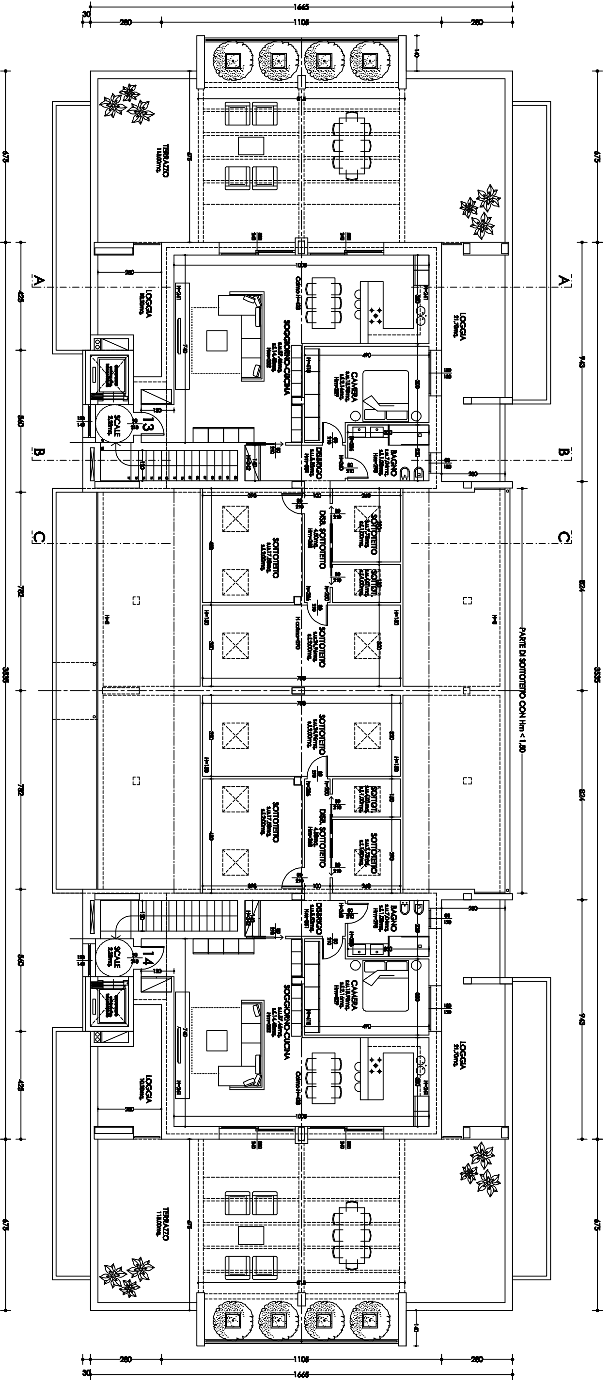
PIANTA PIANO SECONDO Scala 1:100
