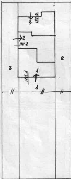
PIANO TERRA CON CORTE ANNESSA
