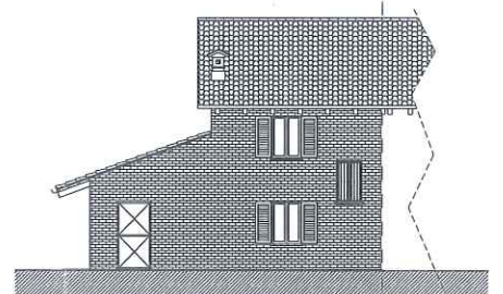
PROSPETTO NORD - 1:100
