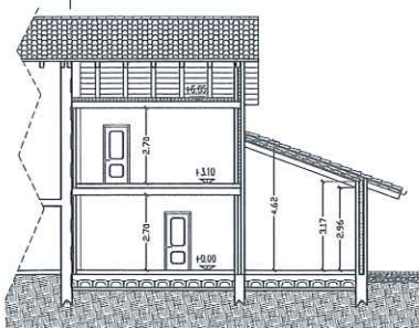
SEZIONE A-A - 1:100
