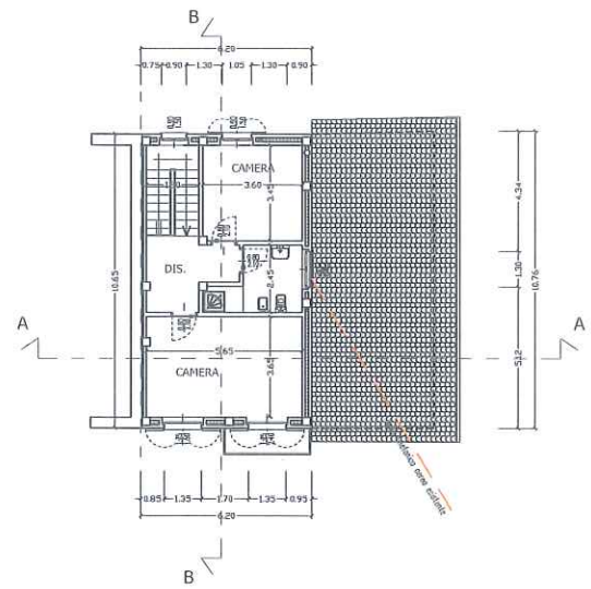
PIANTA PIANO PRIMO - 1:100
