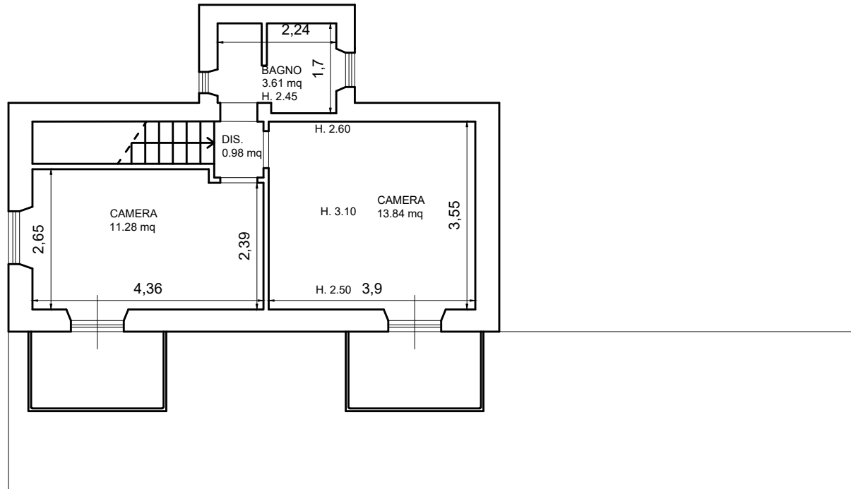
PIANO PRIMO
